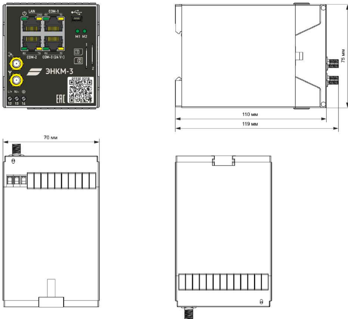
Рисунок 1.5. Габаритные размеры ЭНКМ-3-Х-Х-000
