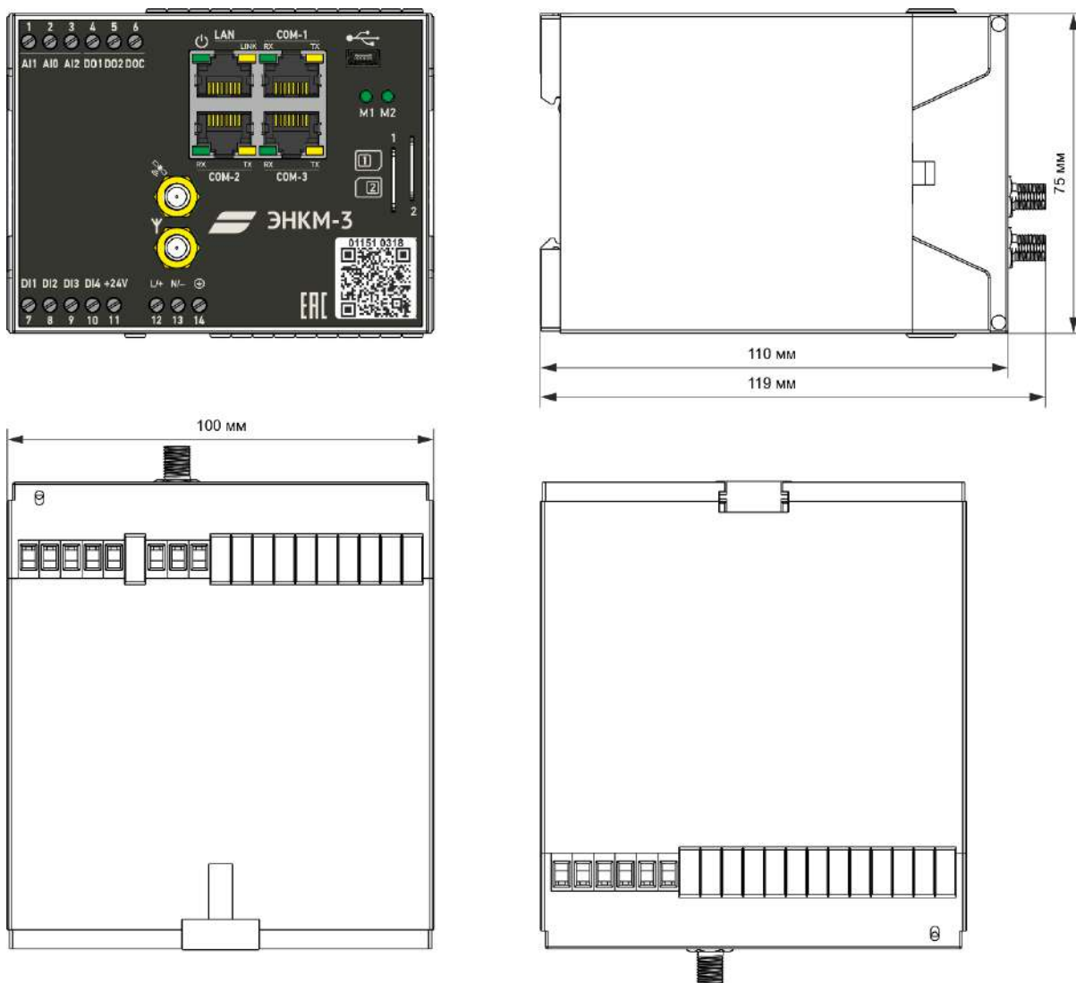
Рисунок 1.6. Габаритные размеры ЭНКМ-3-Х-Х-XXX
